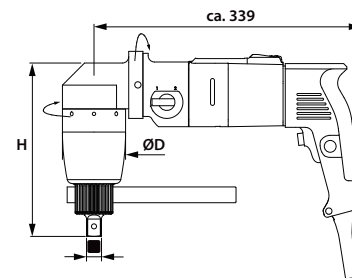
LEW-S elektrická úhlová verze
