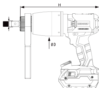
LDA-S verze s baterií
